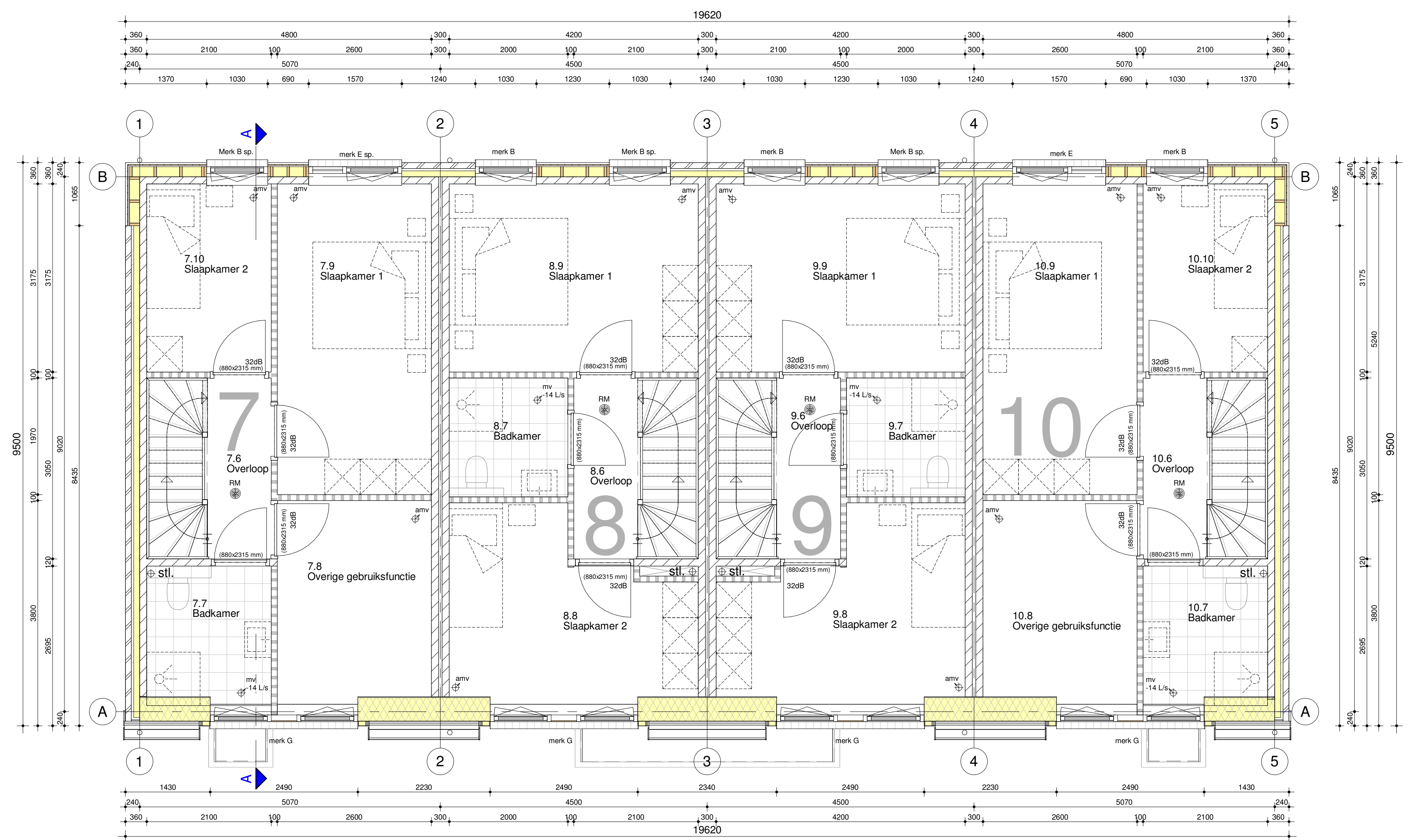
Eerste verdieping (7 t/m 10) (schaal 1 : 50)
