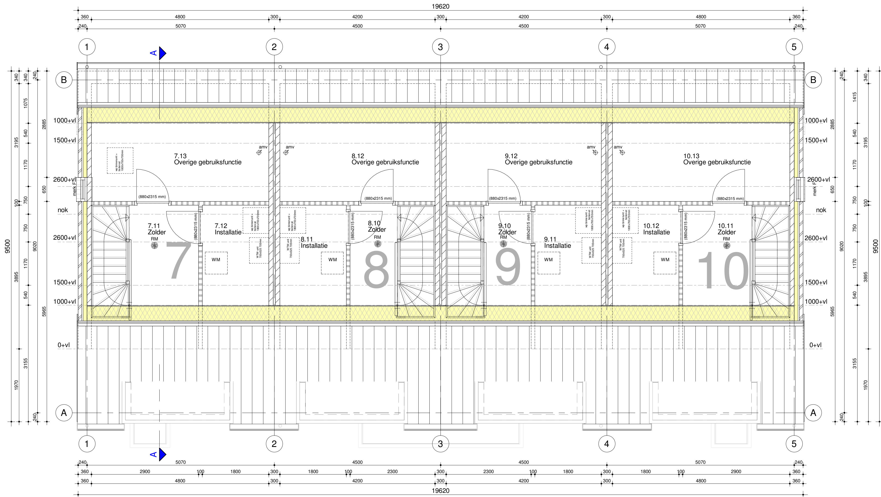
Tweede verdieping (7 t/m 10) (schaal 1 : 50)
