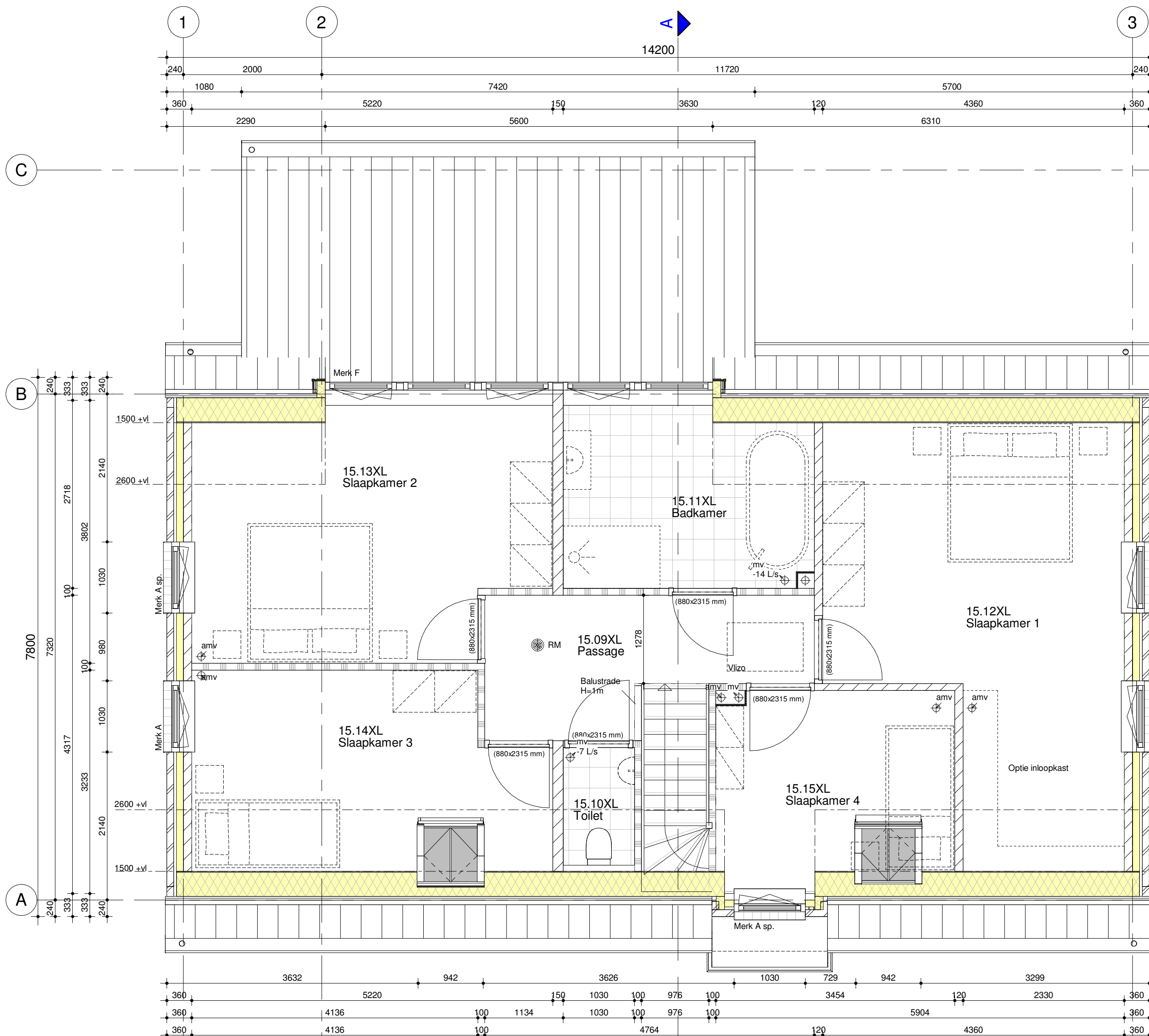
1 Eerste verdieping (schaal 1 : 50)
