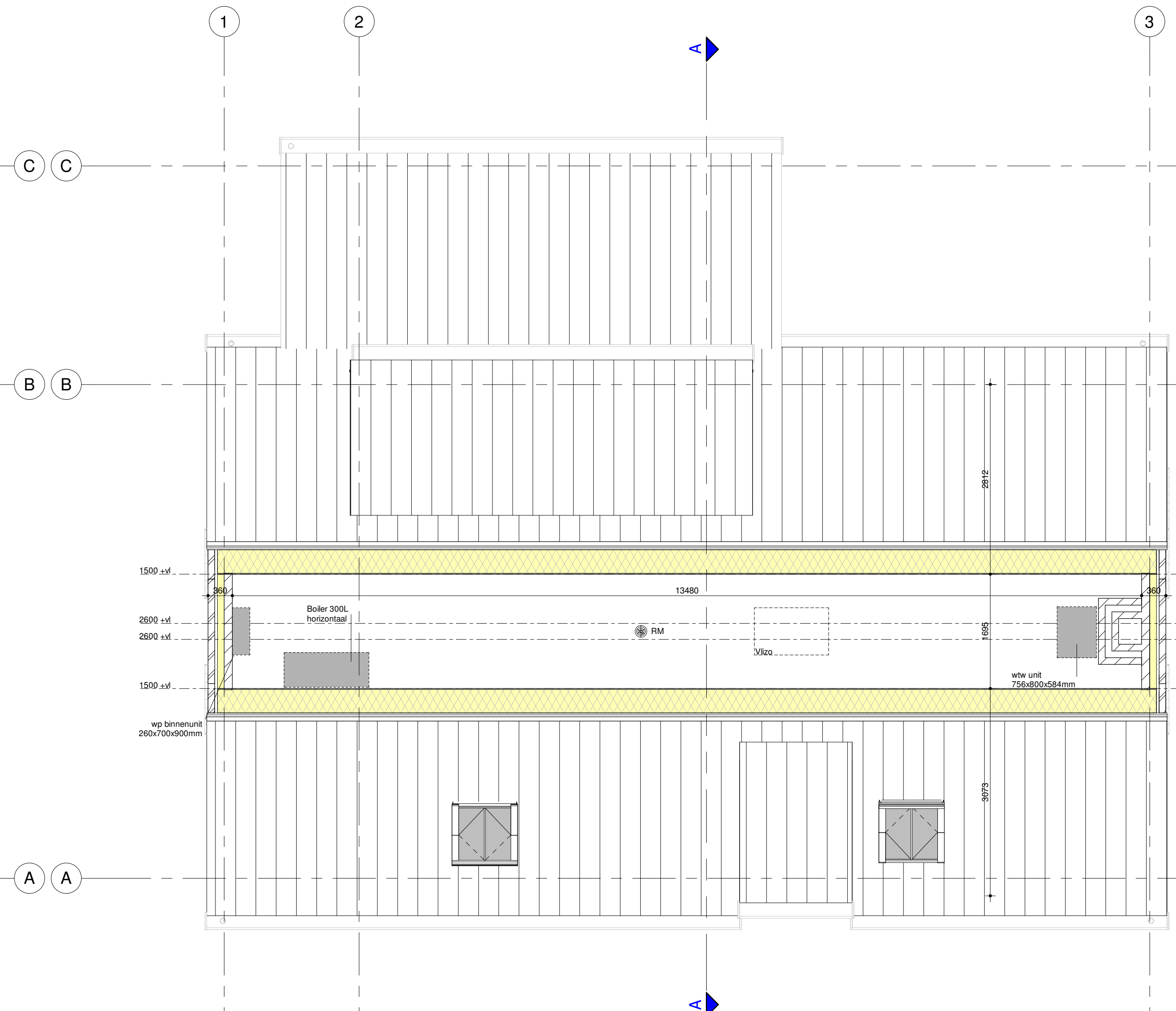
Zolder (schaal 1 : 50)
