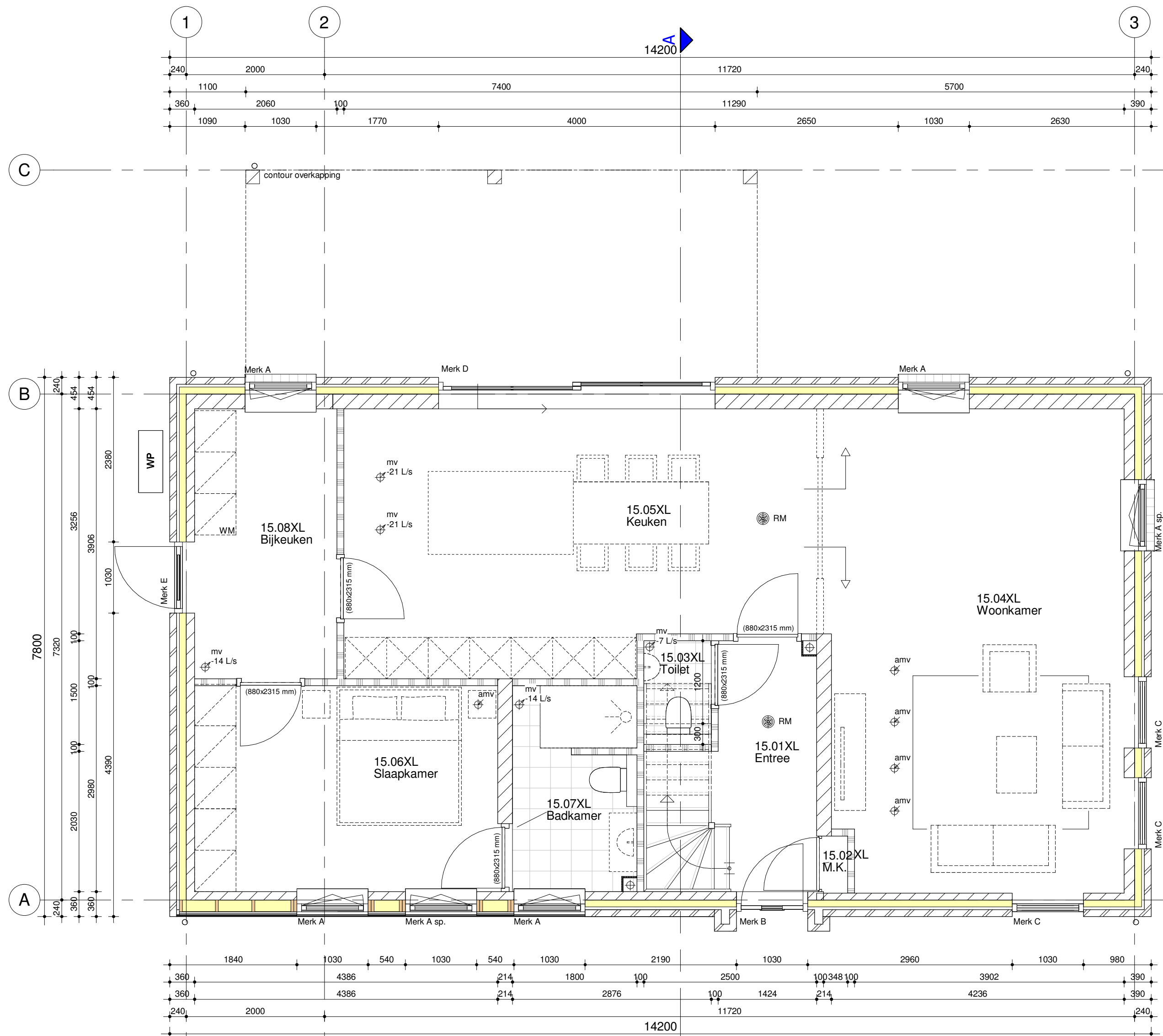
1 Begane grond (schaal 1 : 50)
