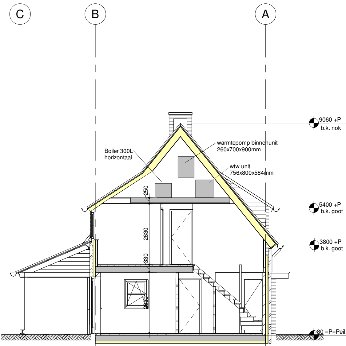
Doorsnede AA' (schaal 1 : 100)
