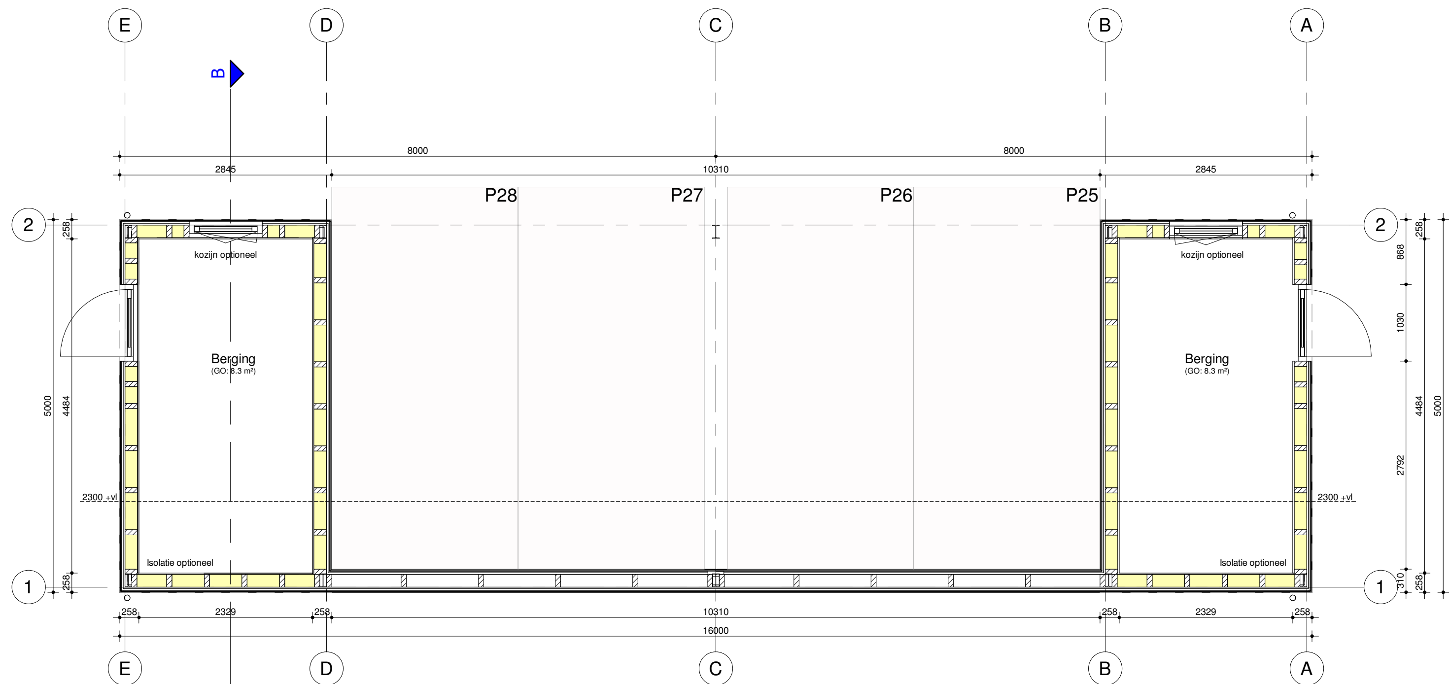
Begane grond berging (schaal 1 : 50)
