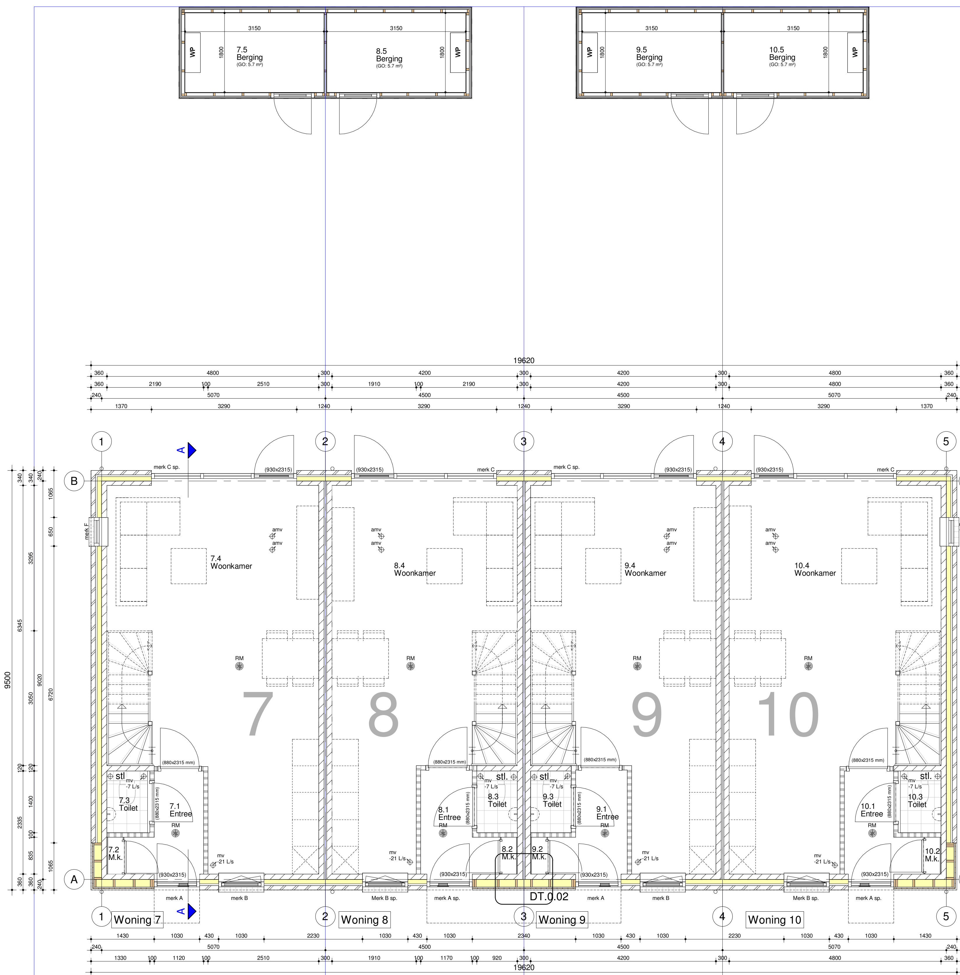
Begane grond (7 t/m 10) (schaal 1 : 50)
