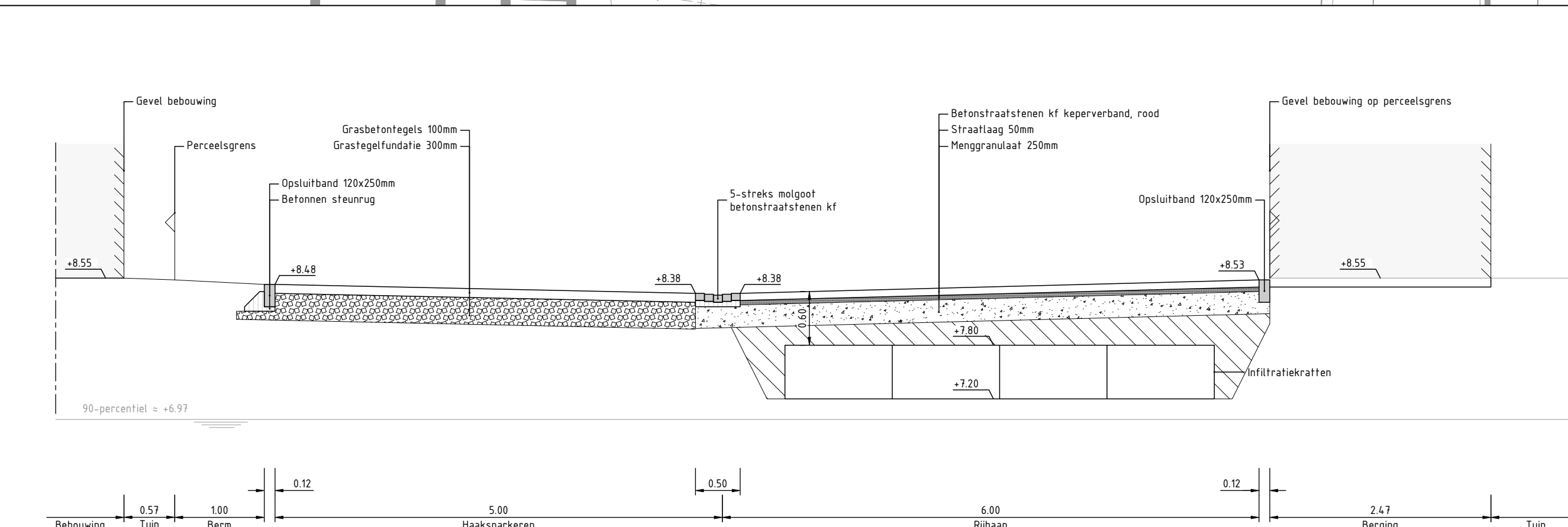
Dwarsprofiel B-B Schaal 1 : 50
