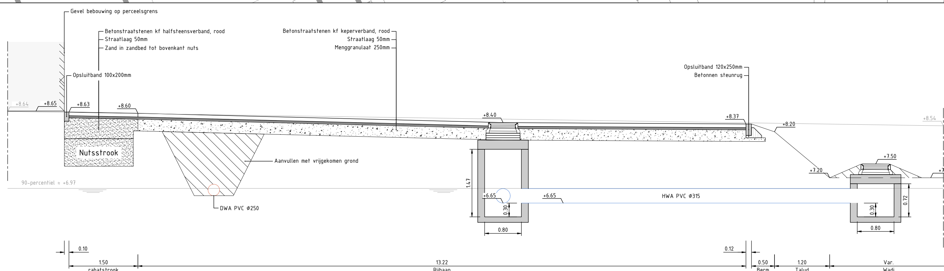
Dwarsprofiel A-A Schaal 1 : 50
