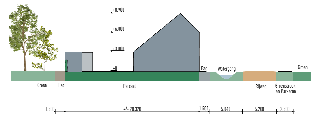
Doorsnede C-C
