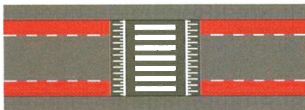
Figuur 4-2: voorbeelden toe te passen maatregelen t.b.v. veilige inrichting VOP's
