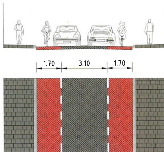
Figuur 2-1: dwarsprofiel
